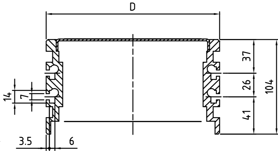
フレーム断面図
